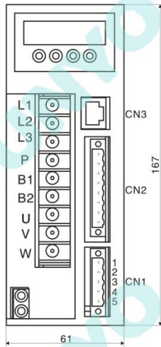
安装尺寸: (长)167mm × (宽)61mm × (高)151mm
