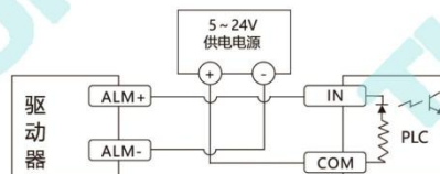
将输出ALM接成sinking型输出,与PLC的输入相连
